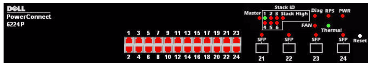
Εικόνα 1-3. PC 6224P
